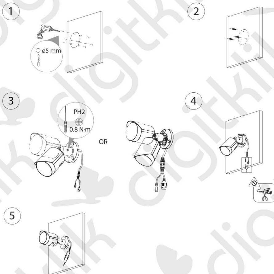
Slika 3-3 Kabel, ki gre skozi stranski kabelski jašek
