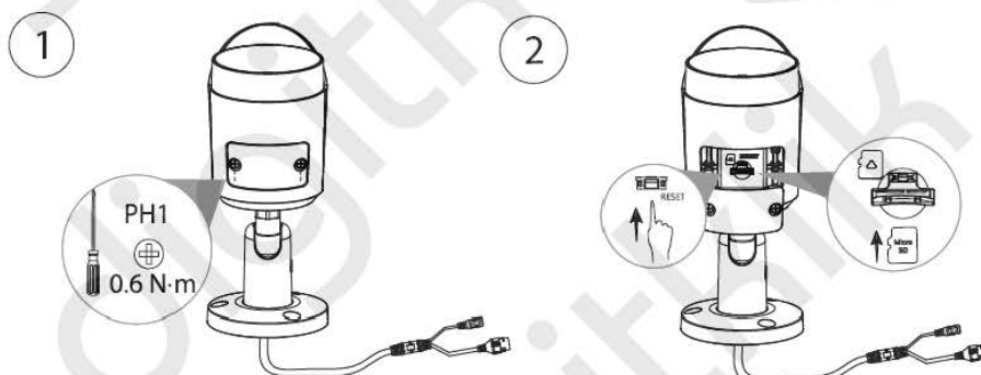
Slika 3-2 Namestitev SD kartice
