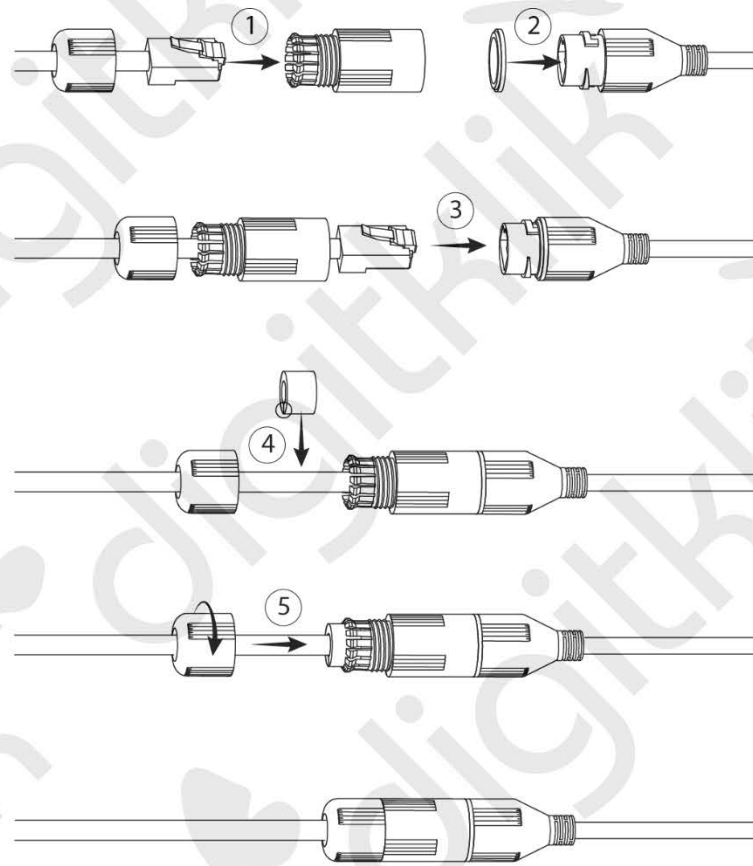
Slika 3-6 Namestitev vodotesnega priključka
