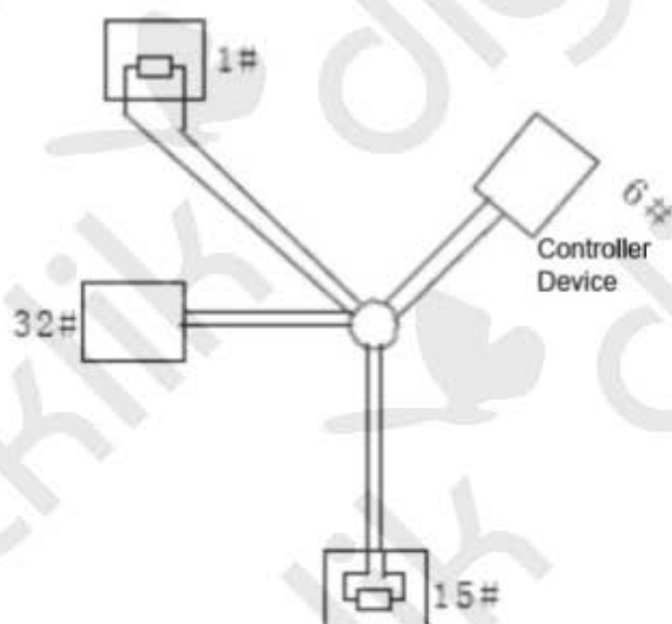
Slika 3-1 Običajen način povezovanja naprav
